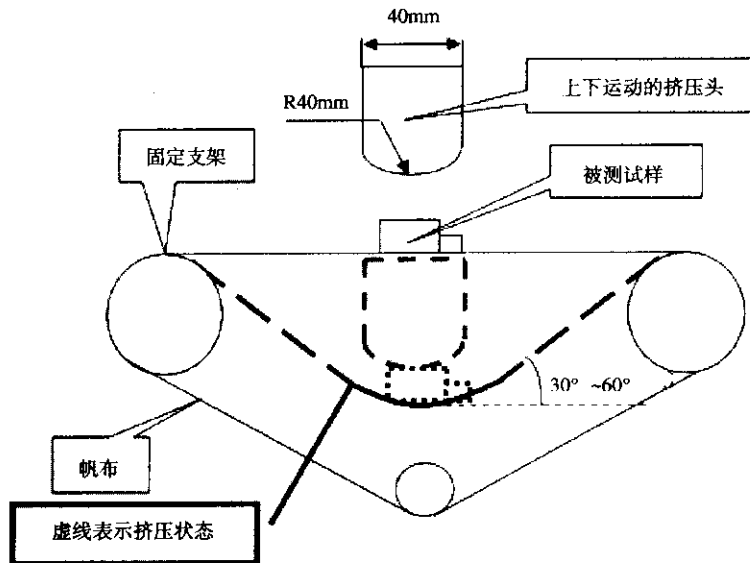
图1 挤压测试的结构
