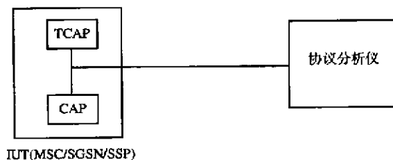
图 1 测试结构
