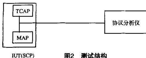
图2 测试结构
