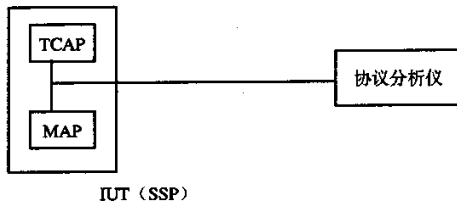
图 1 测试结构
