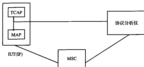
图3 测试结构
