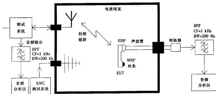
图 1 音频校准的电路配置
